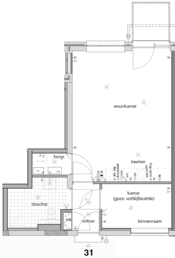
Eerste verdieping
