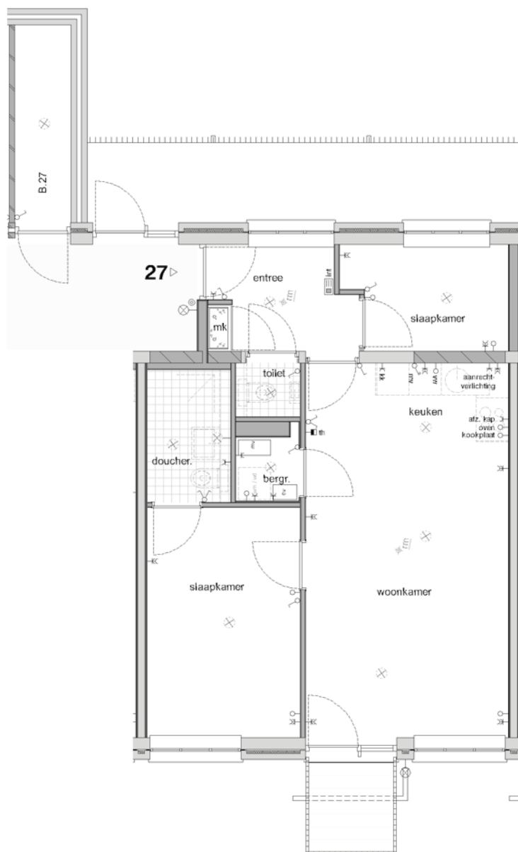
Eerste verdieping
