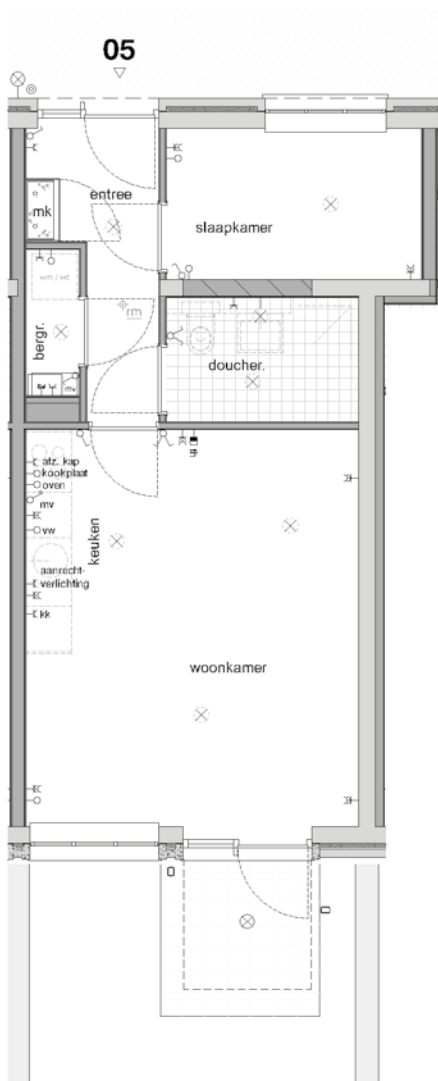
Begane grond
