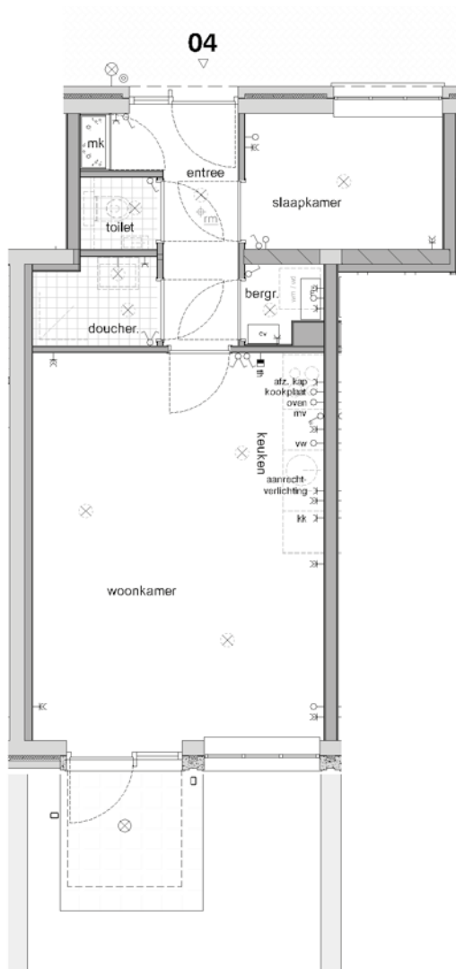
Begane grond
